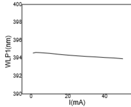
图 4 峰值波长 VS 正向电流
