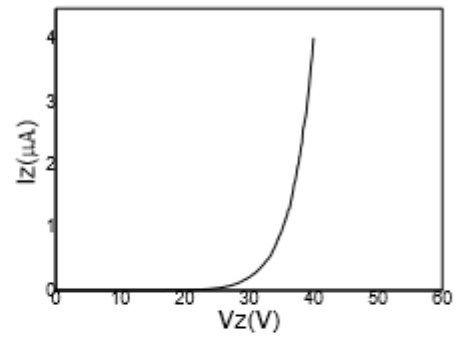
图 2 反向电流 VS 反向电压
