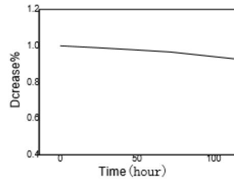
图 6 老化图-裸芯无散热 ( I_f=30\text{mA} , T=22^\circ\text{C} )
