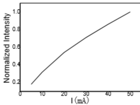
图 5 归一化强度 VS 正向电流
